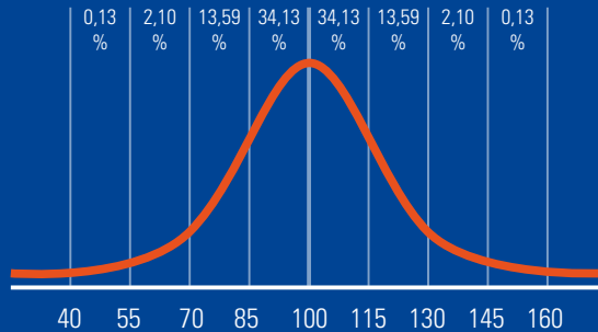
Normalverteilung des Intelligenzquotienten
